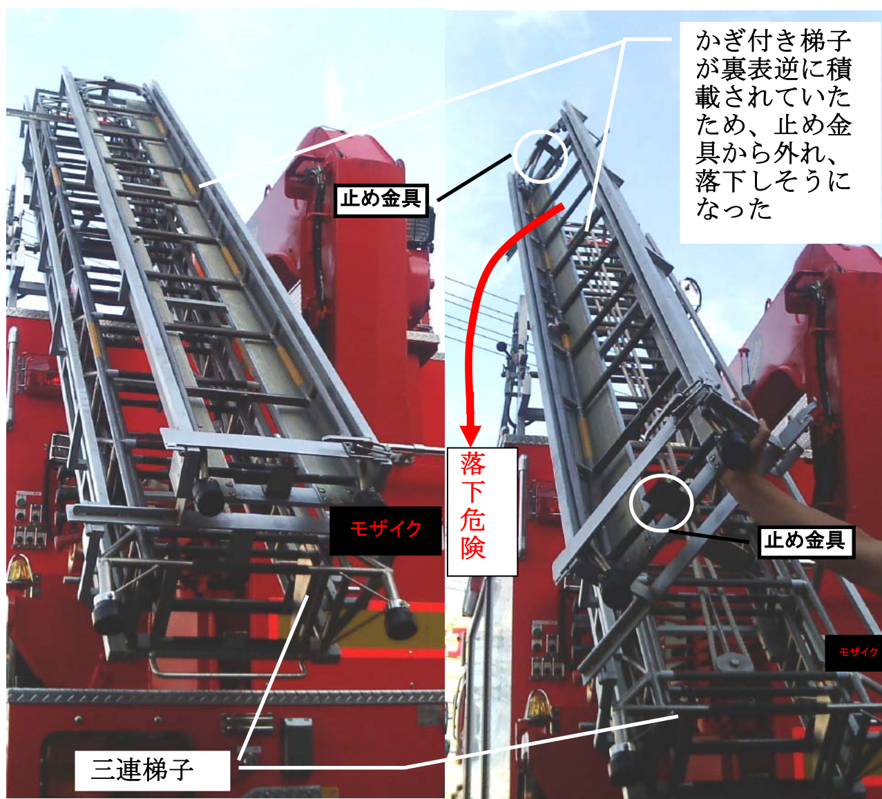
①三連梯子（かぎ付き梯子）積載状況
