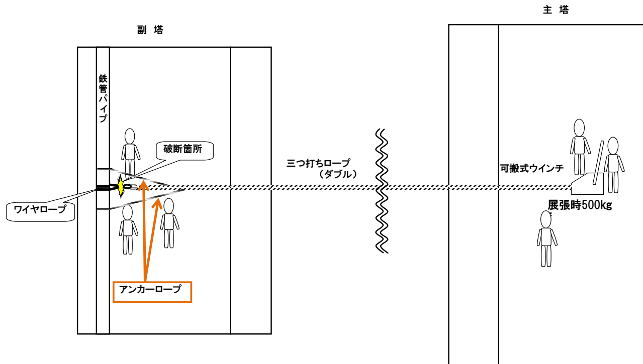
ヒヤリハット事例(ワイヤロープを支点としたロープ展張時の破断事例)
