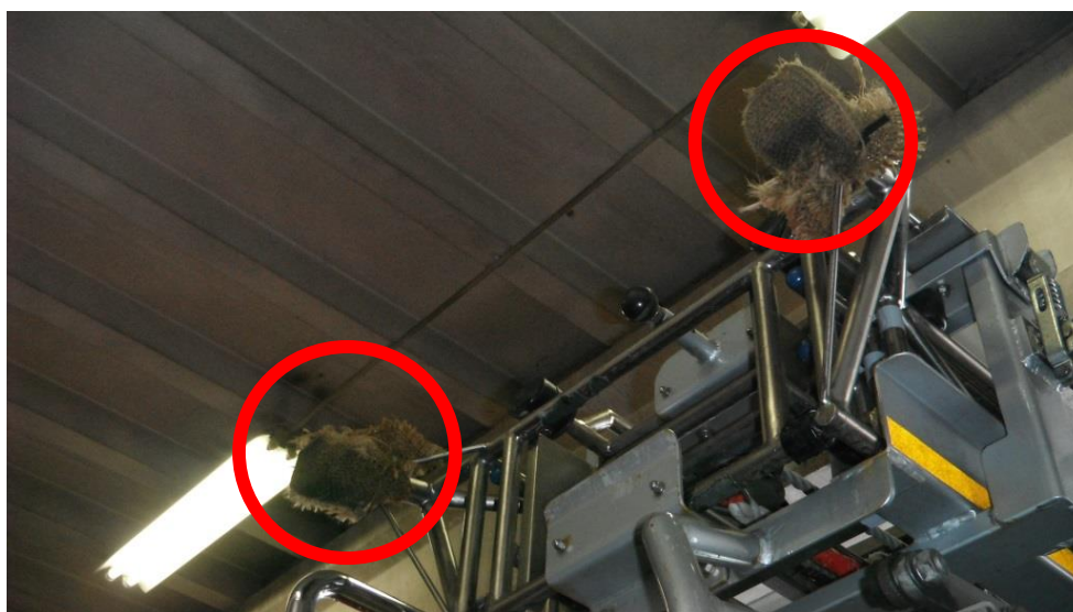
○冬期間の三連はしご基底部の滑り防止を図るため、麻袋を三連はしご基底部ゴムに装着
