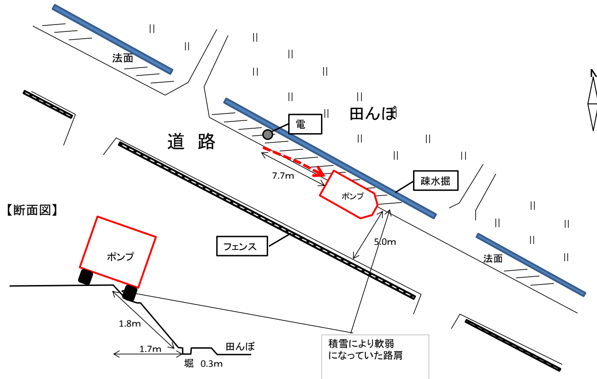
ポンプ車脱輪状況図
