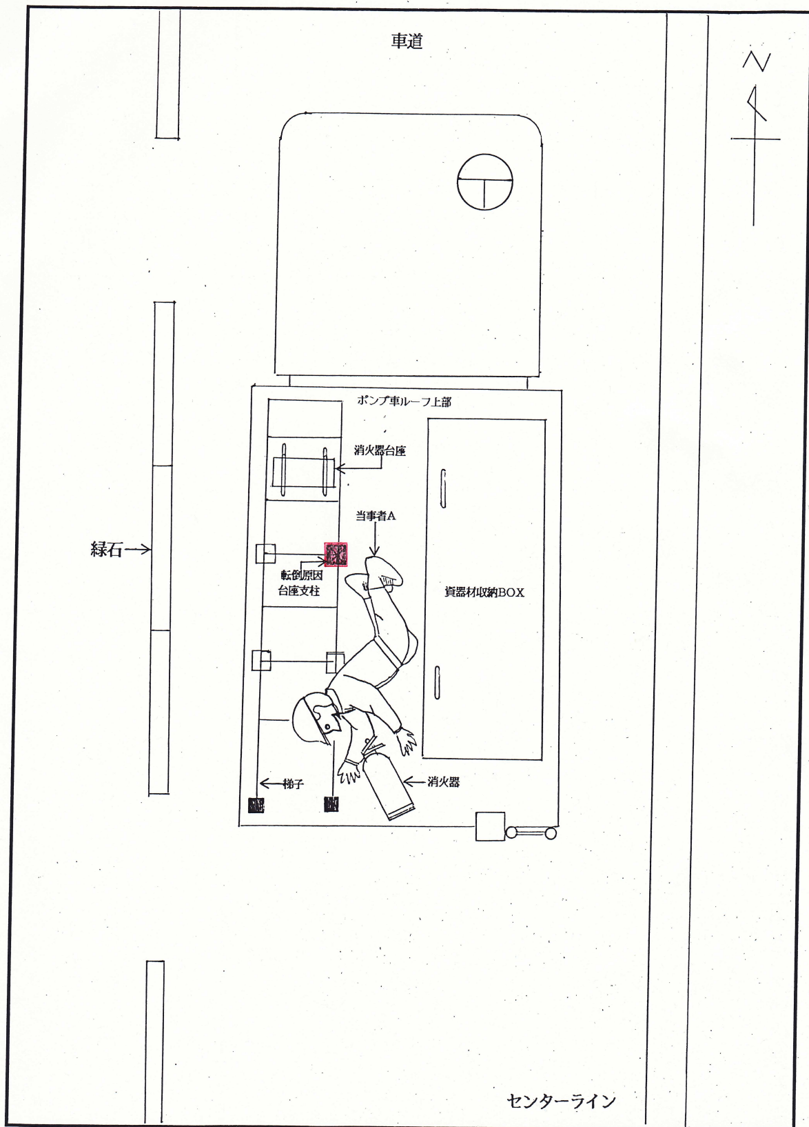
ポンプ車ルーフ上部図
