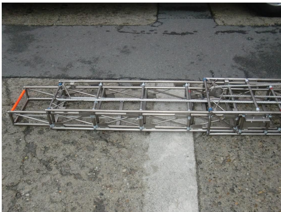
三連はしごの2連目、3連目同時伸てい状況の部分拡大（再現）
