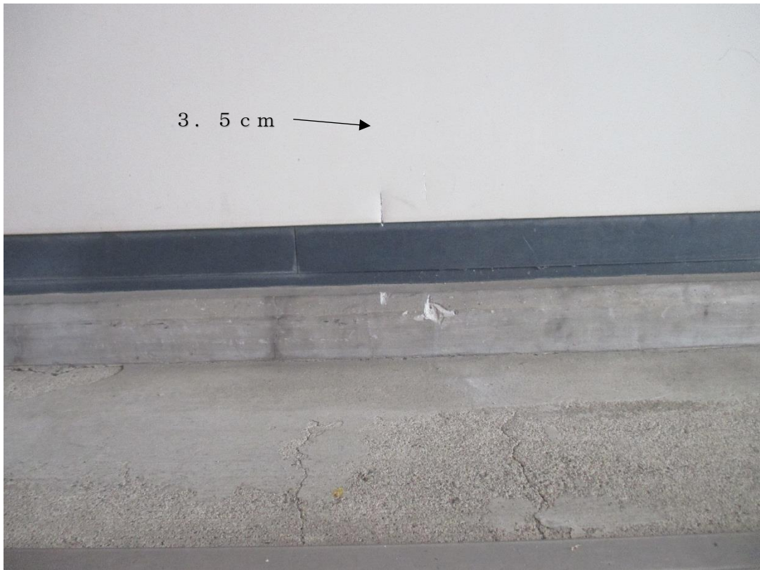
外壁及び基礎コンクリートの破損状況
